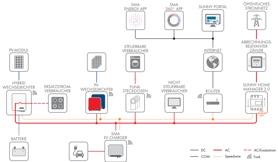
Abbildung 5: Aufbau des Systems
