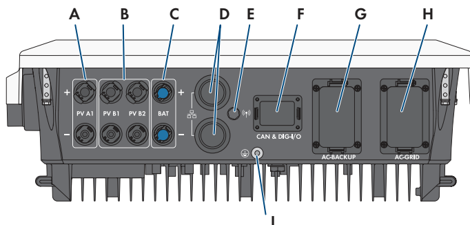
Abbildung 13: Anschlussbereiche an der Unterseite des Wechselrichters
