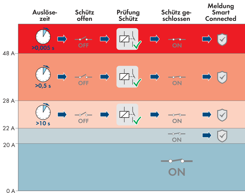
Abbildung 22: Verhalten des Schützes zwischen AC-Ersatzstromanschluss und Anschluss an das öffentliche Stromnetz bei erhöhter Stromstärke
