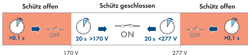
Abbildung 23: Verhalten des Schützes zwischen AC-Ersatzstromanschluss und Anschluss an das öffentliche Stromnetz bei zu hoher oder zu niedriger Spannung
