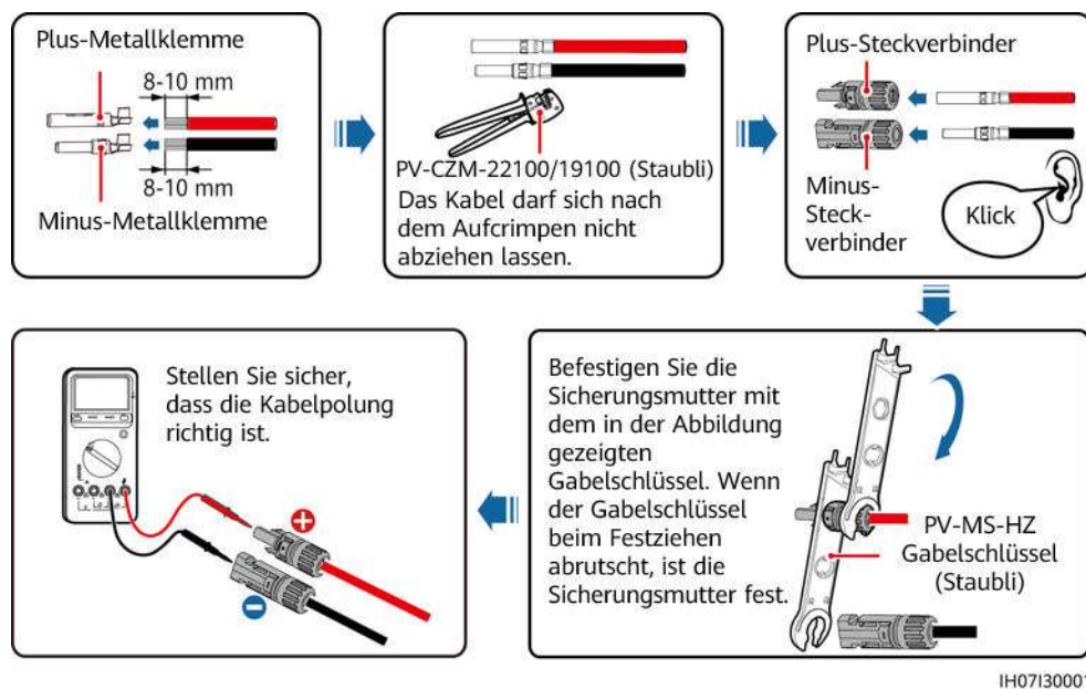
Abbildung 5-13 Anschließen der DC-Eingangsstromkabel
