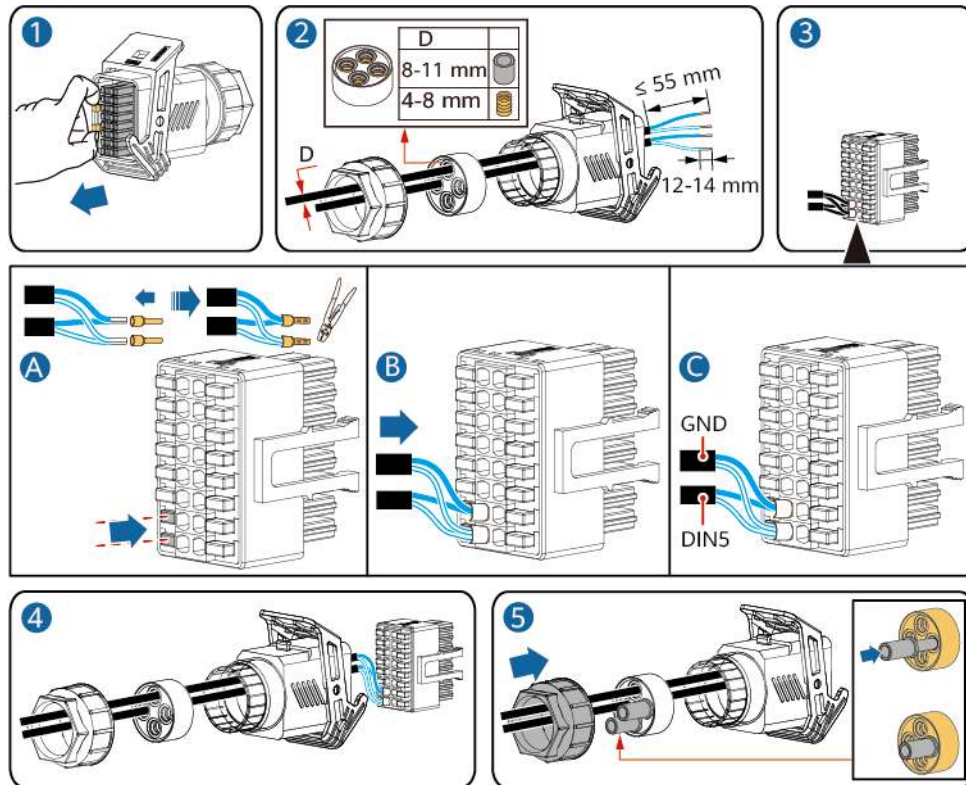
Abbildung 5-39 Kabelmontage
