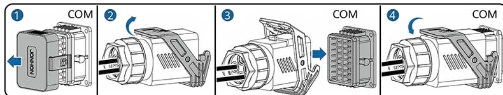
Abbildung 5-40 Sichern des Signalkabelanschlusses
