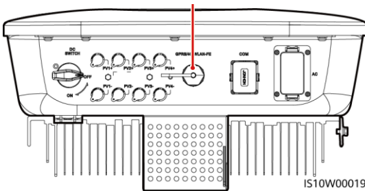
Smart Dongle-Anschluss (GPRS/4G/WLAN-FE)
