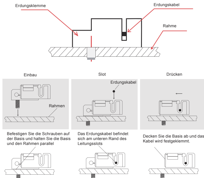
Abbildung 11 Installationsmethode der Erdungsklemme
