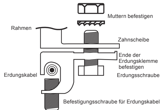
Abbildung 12 Installationsmethode der Erdungsschraube
