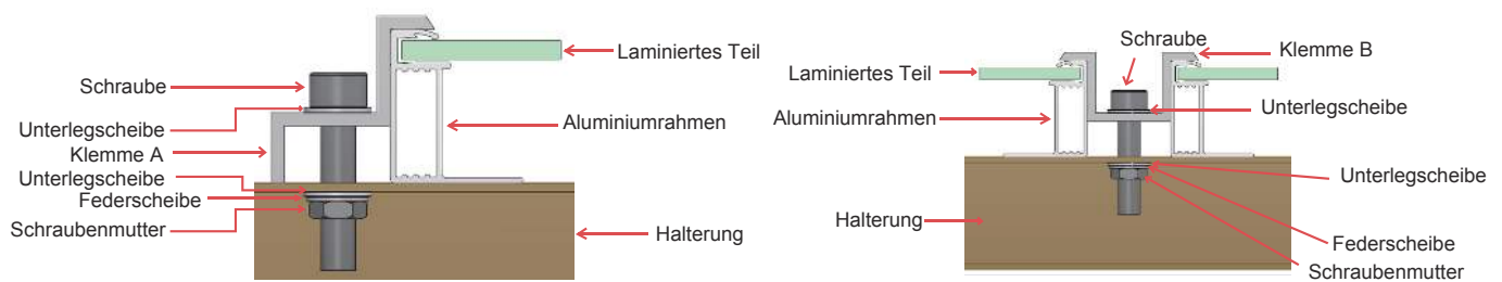
Abbildung 5 Klemminstallation des Monofacial-Moduls
