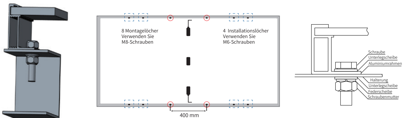
Abbildung 4 Bolzeninstallation von Monofacial-Modulen
