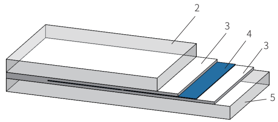
Bifacial-Doppelglasmodul (Rahmenlos)
